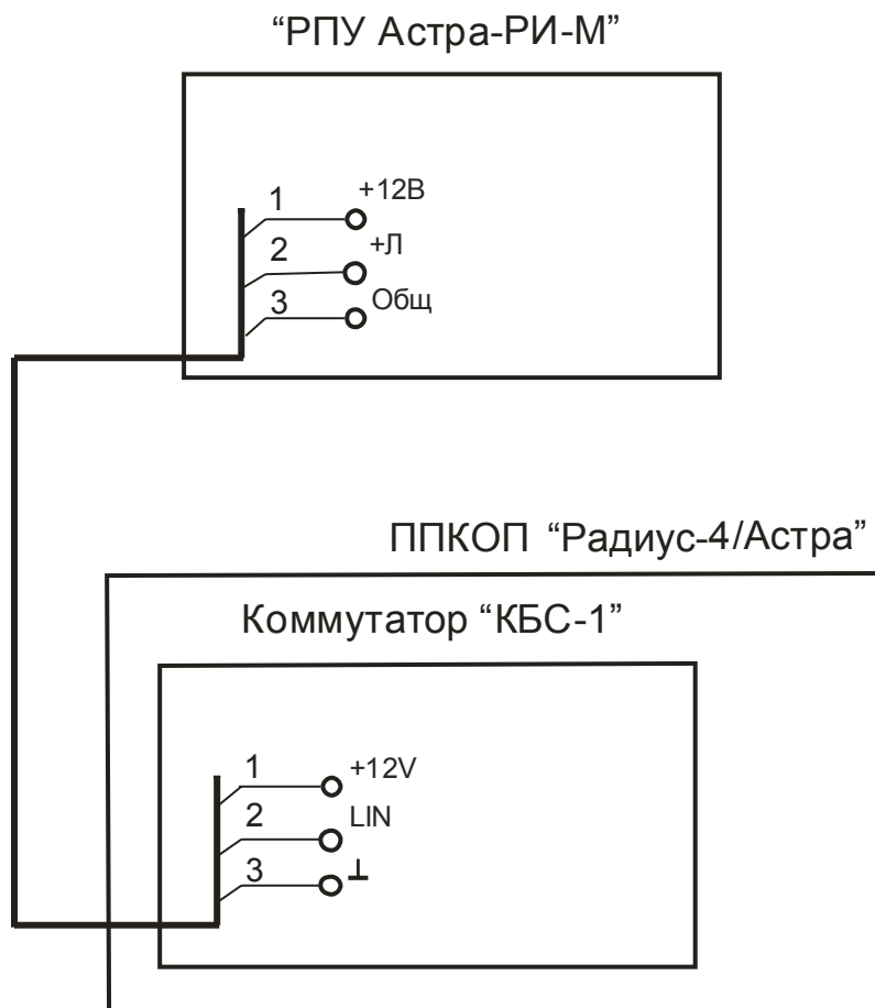
Рисунок 5 – Схема подключения РПУ к коммутатору при программировании
