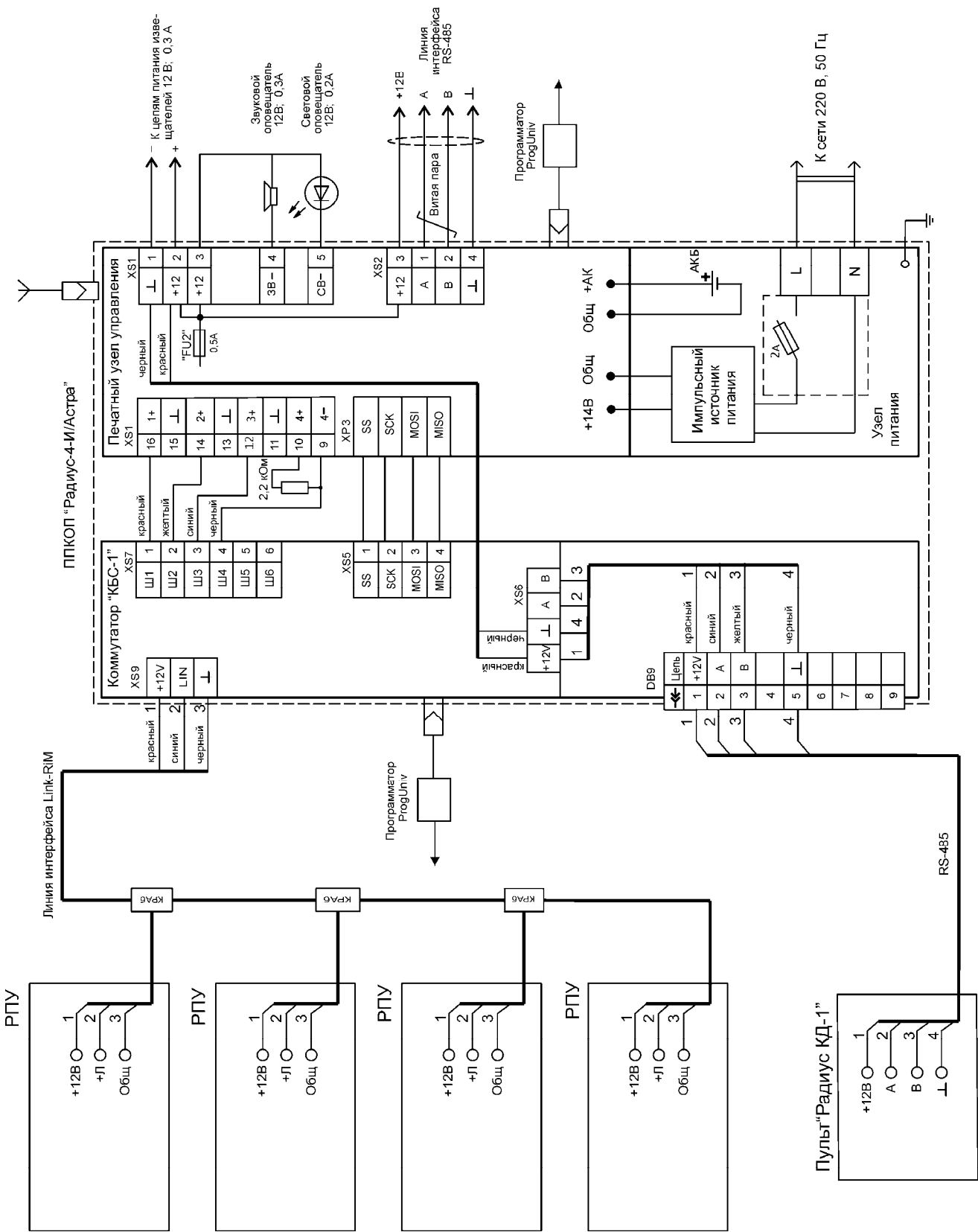
Схема подключения ППКОП "Радиус-4/Астра"
