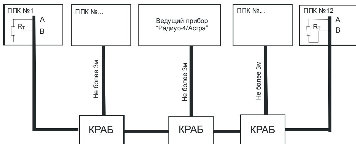
Вариант 2 - двухлучевой
