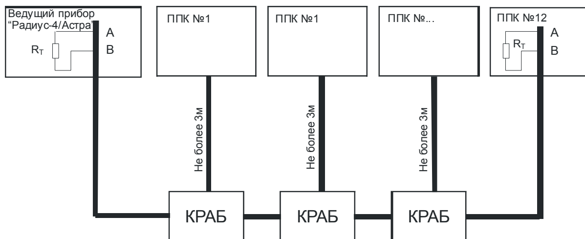
Вариант 1 -однолучевой
