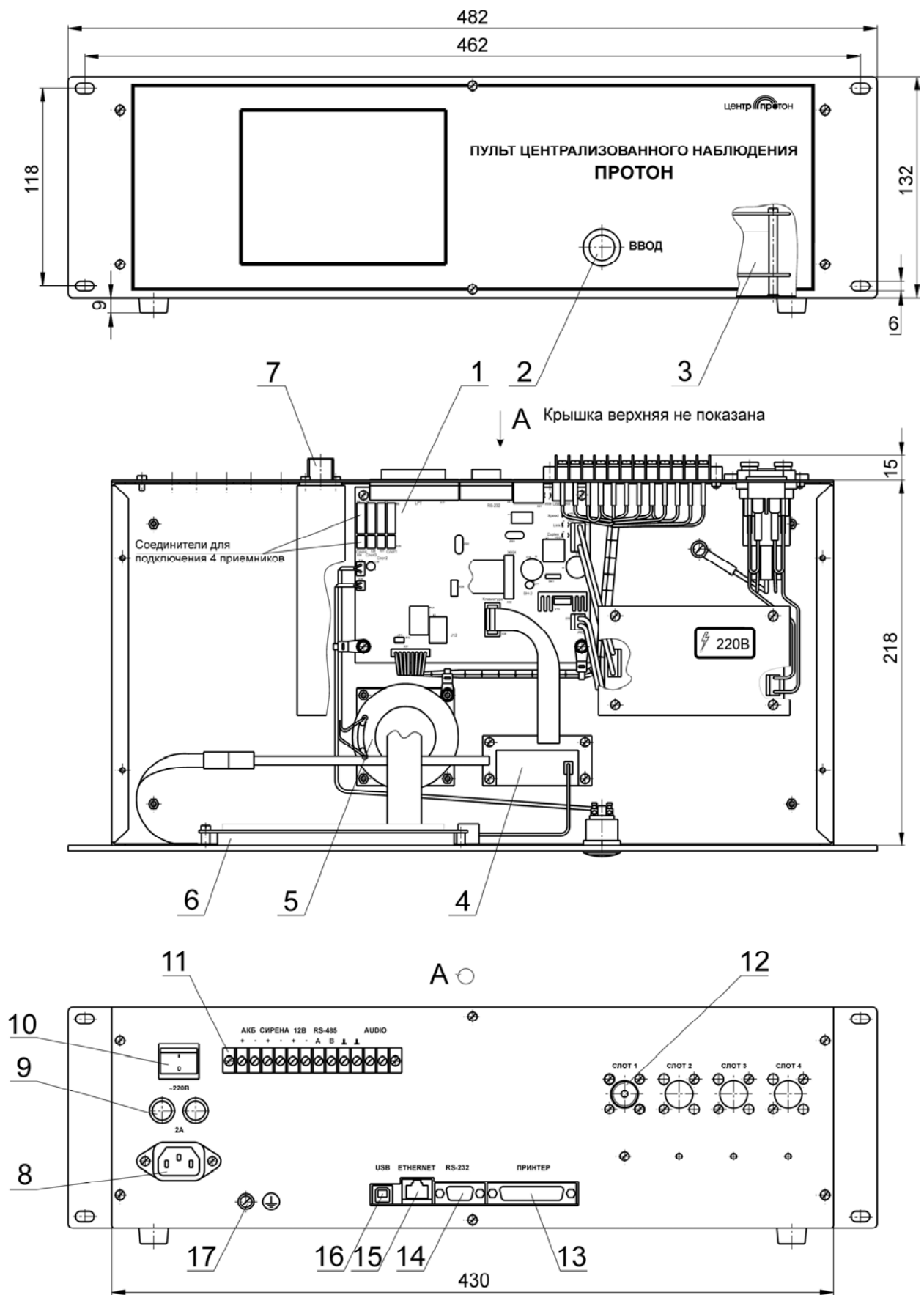
Рисунок 1 – ПЦН «Протон»
