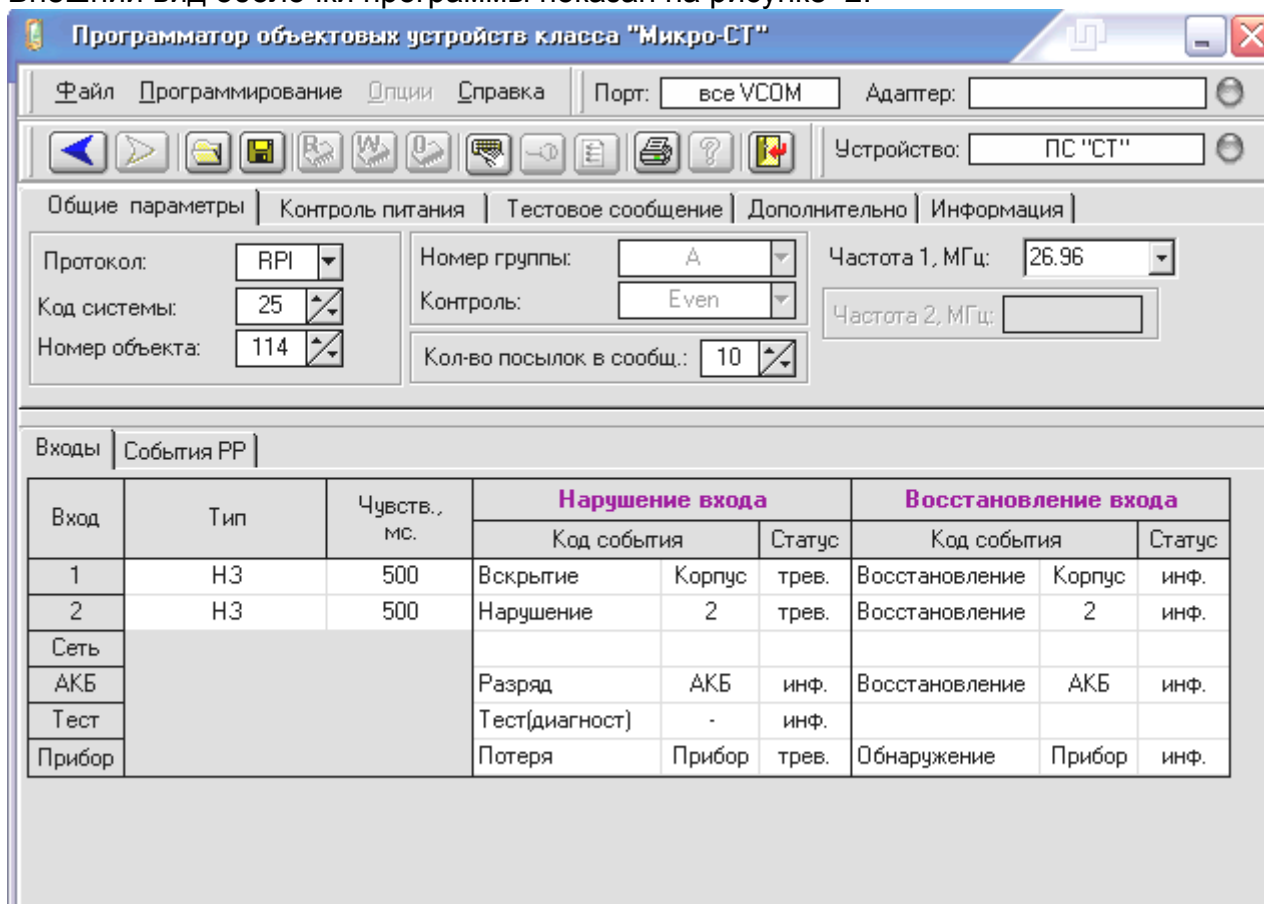
Рисунок 2 – Внешний вид оболочки программы ProgProton
