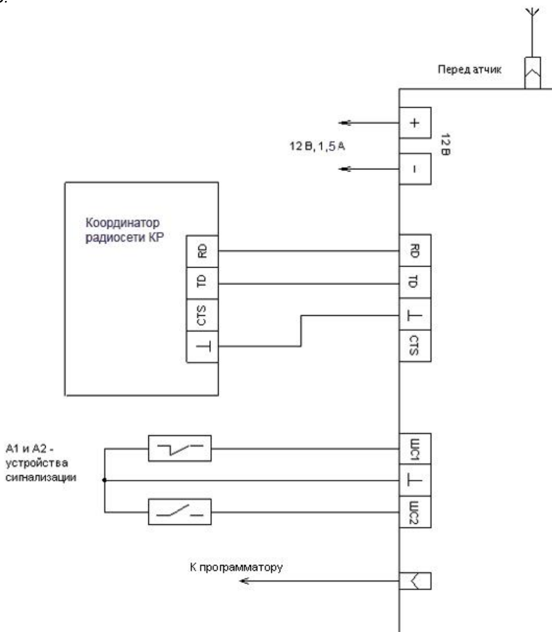
Рисунок 4 – Схема подключения передатчика «СТ»
