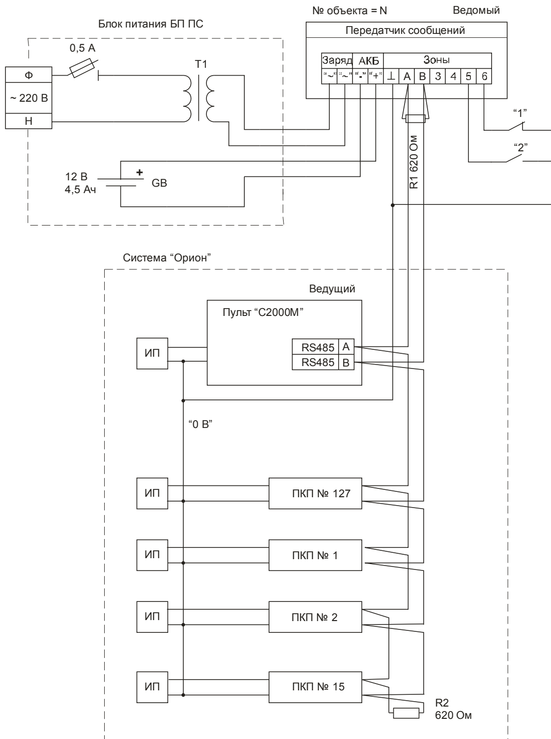
Рисунок 4 – Схема подключения передатчика
