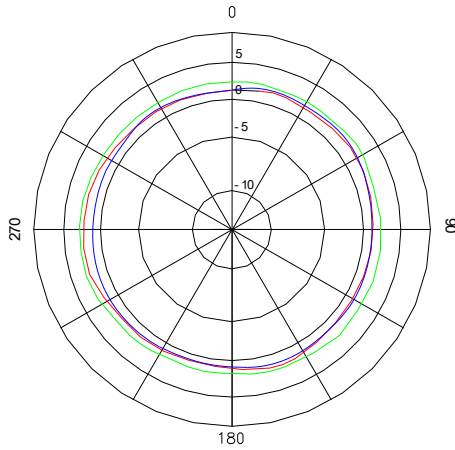
水平面方向图(2.4G天线) Horizontal Pattern
